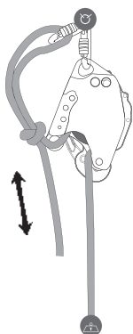
Рис 8 Системы подъёма вручную
