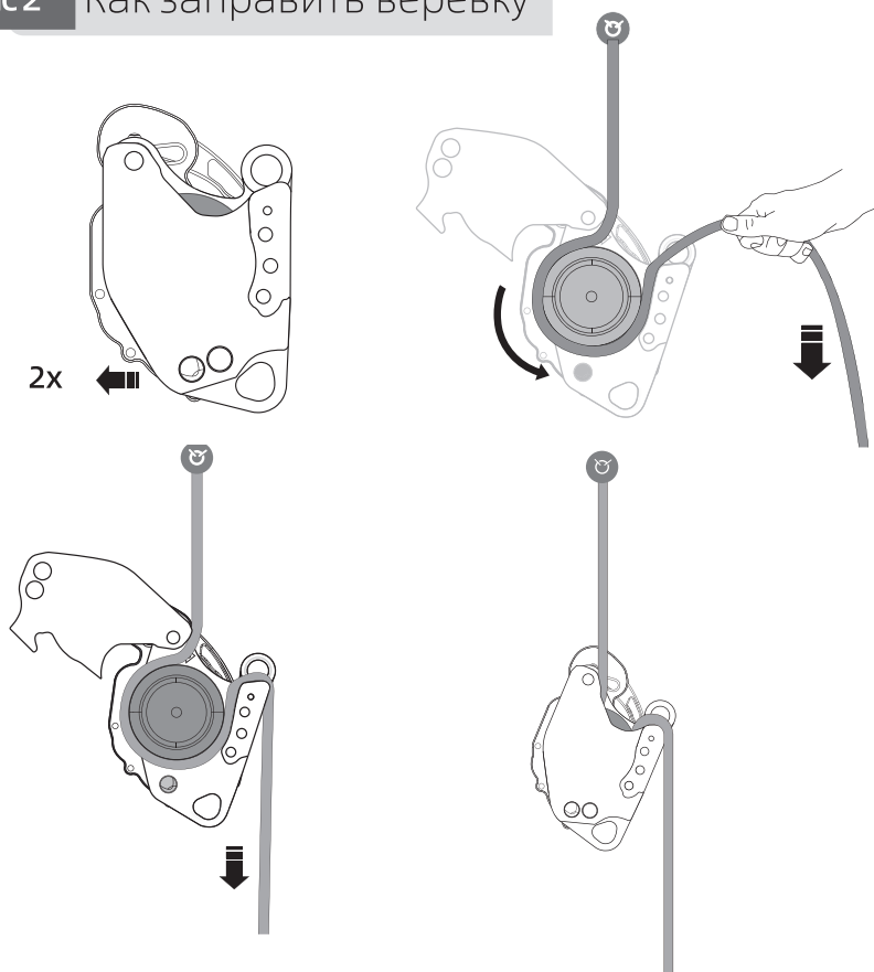
Рис 2 Как заправить верёвку
