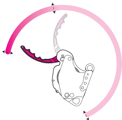
Рис 2 Как заправить верёвку
