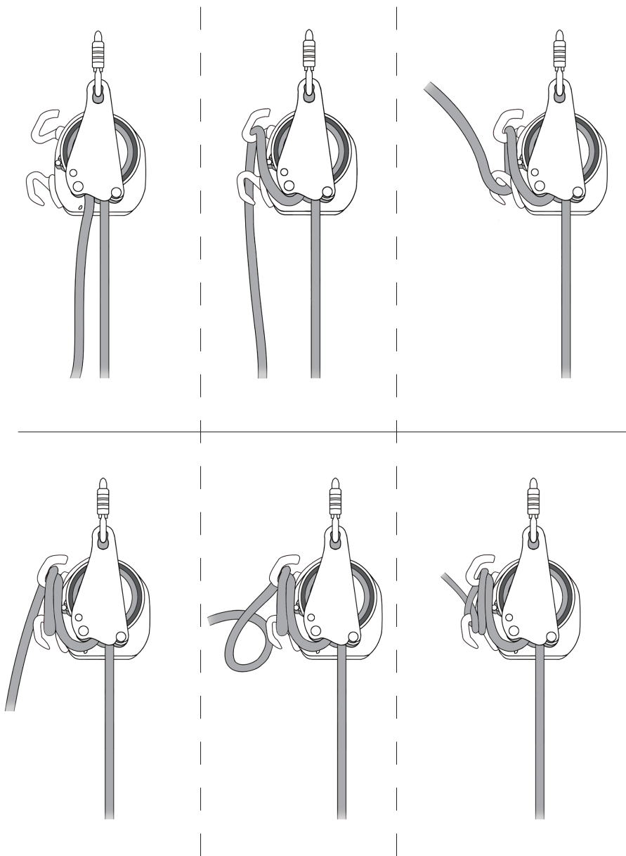
Рис 8 Фиксация верёвки
