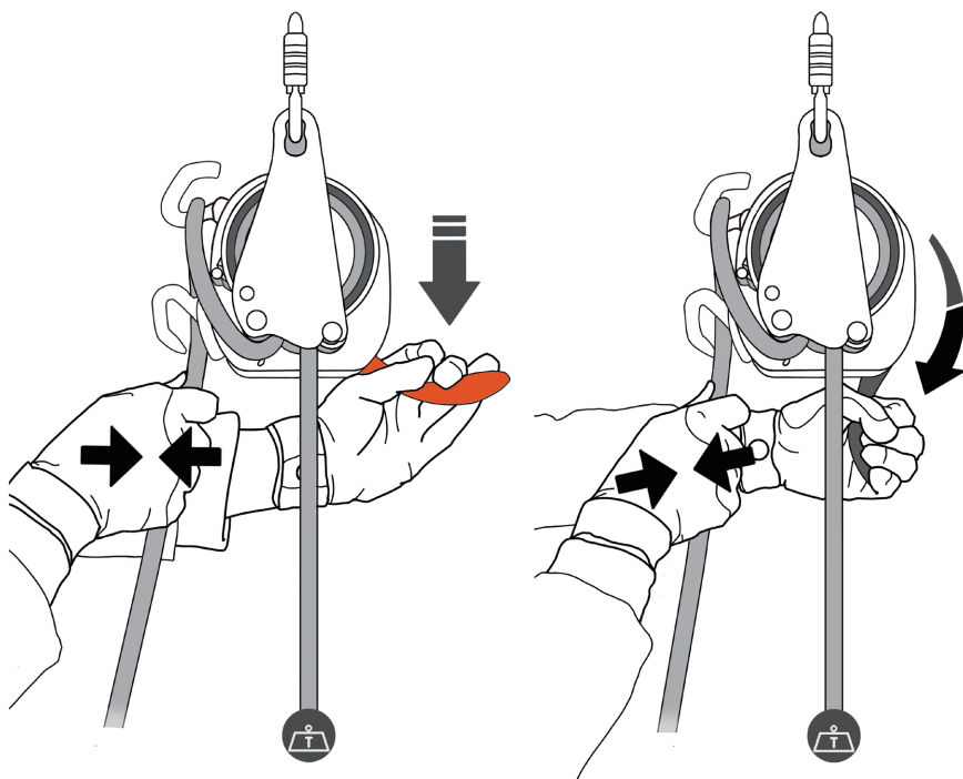
Рис 5 нормальный спуск
