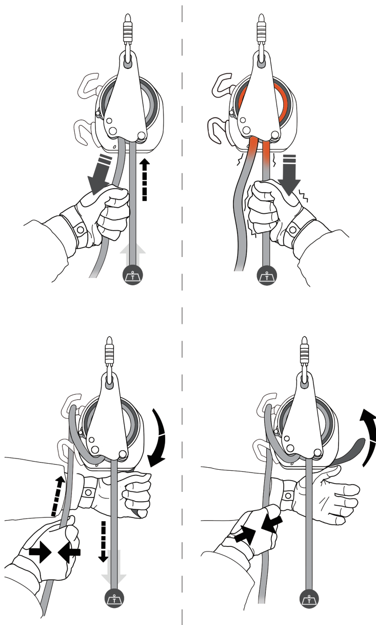
Рис 4 функциональная проверка
