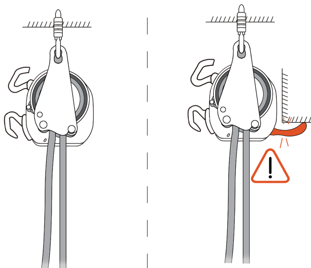
Рис 9 Обеспечьте свободный ход рукояти.
