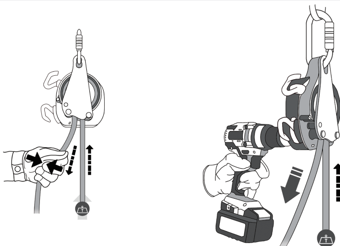
Рис 7 подъём вручную и подъём с шуруповёртом
