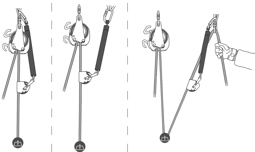
Рис 10 необходимо использовать с резервной системой (Z2 и Z2-R)
