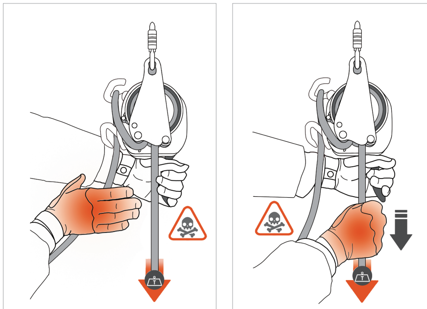
Рис 6 Как не надо придерживать руками верёвку
